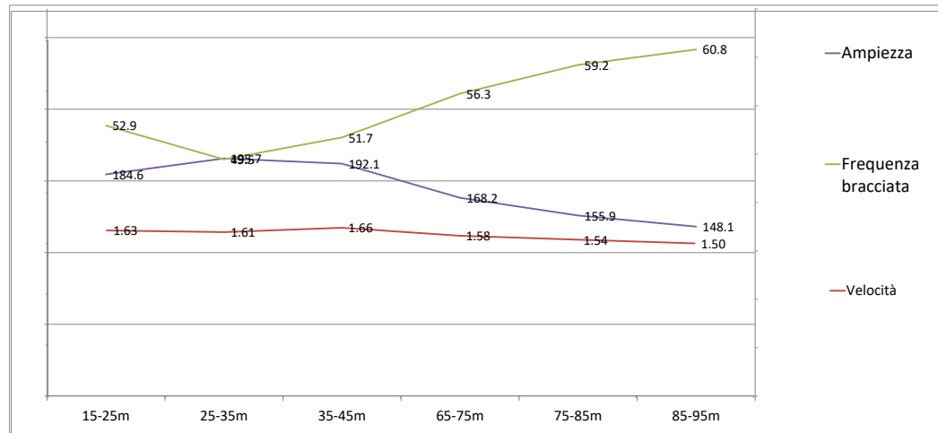
Grafico confronto Ampiezza - Frequenza - Velocità
