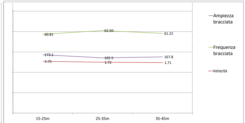
Grafico confronto Ampiezza - Frequenza - Velocità
